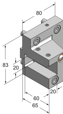
Drehhalter Turning holder WT 150-102
