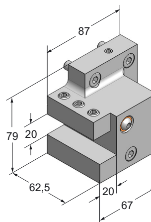
Drehhalter Turning holder WT 100-102
