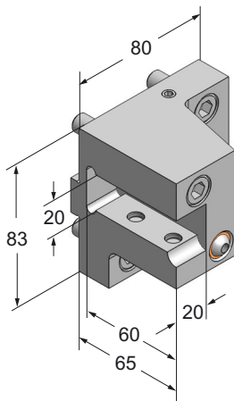
Drehhalter Turning holder WT 150-101
