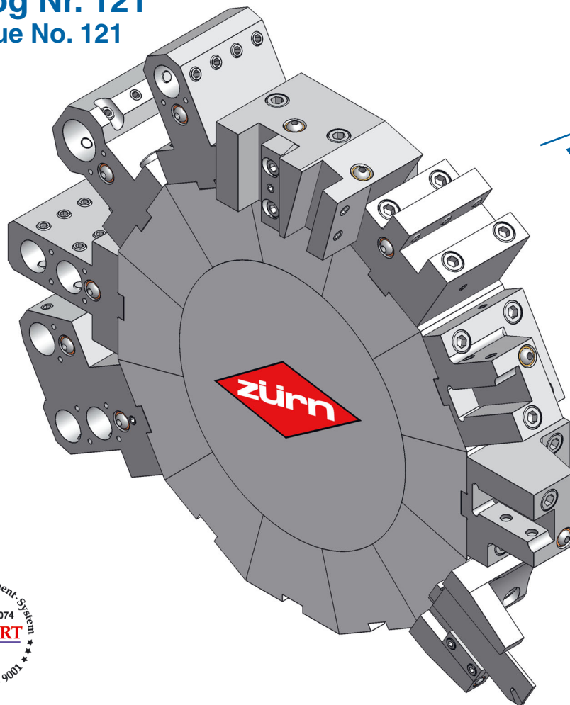
Drehhalter Turning holder WT 100-102
